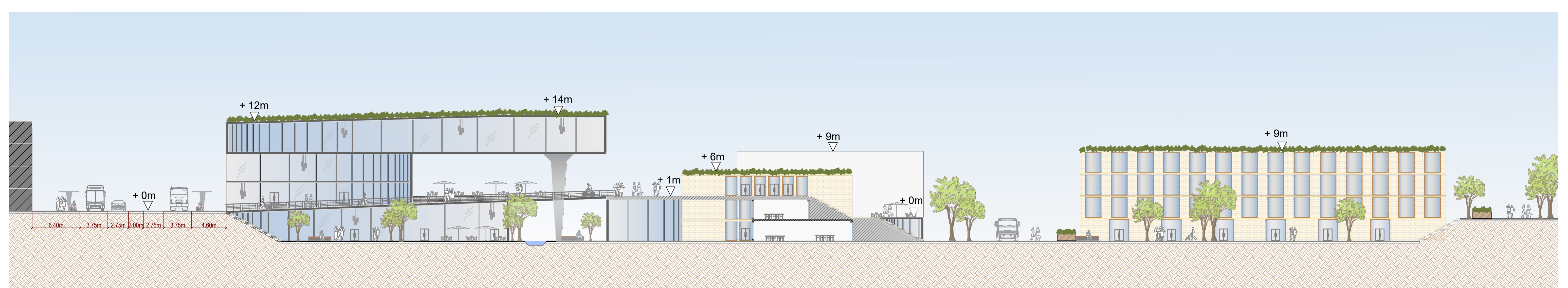
Schnitt AA
