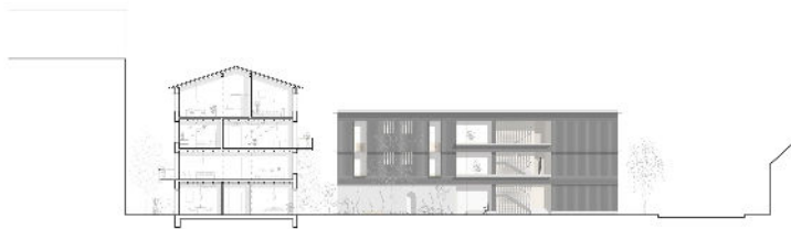
Schnitt II 1:500
