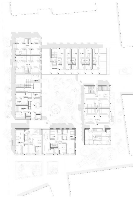
Grundriss/Übergangsplan 1:200
